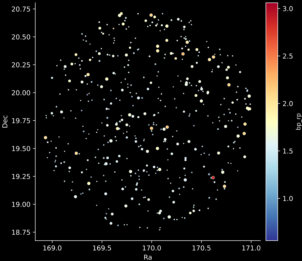
GALAH DR4 Field: [6787] Stars: 463
