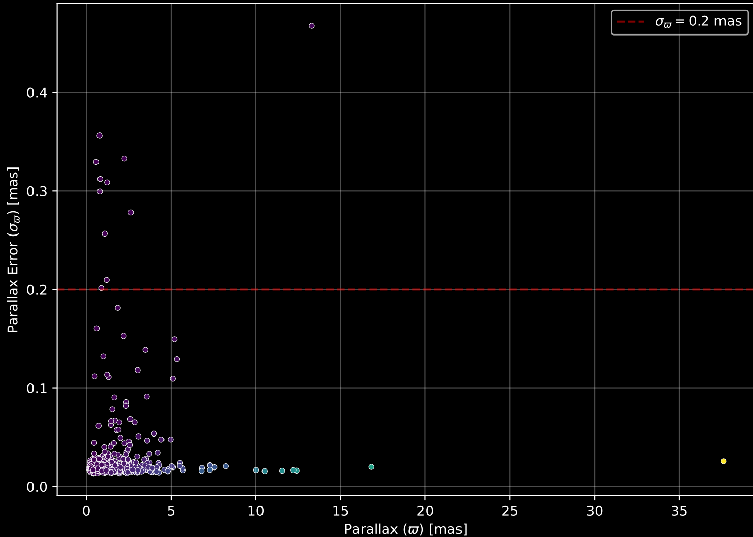
GALAH DR4 Field: [6787] Parallax Quality (n= 463)
