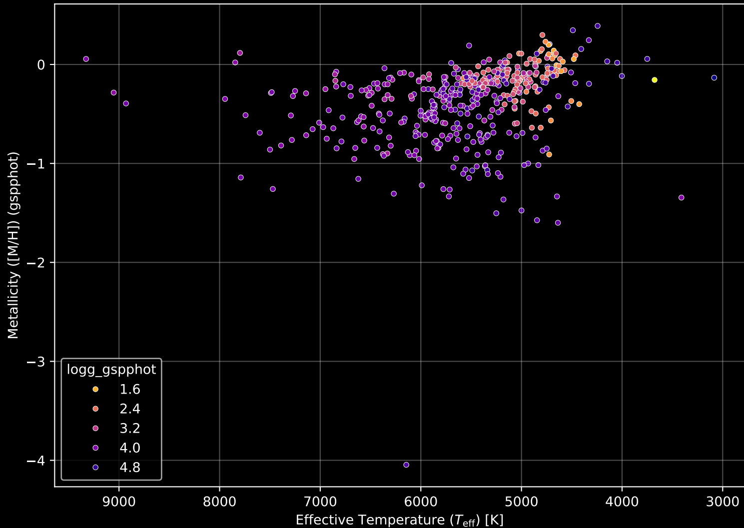
GALAH DR4 Field: [6787] Stellar Population Parameters (n= 463)
