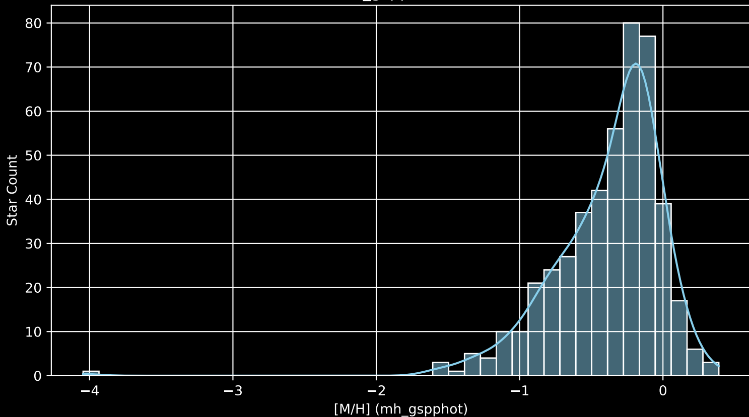
GALAH DR4 Field: [6787] [M/H] (mh_gspphot) (n= 463)
